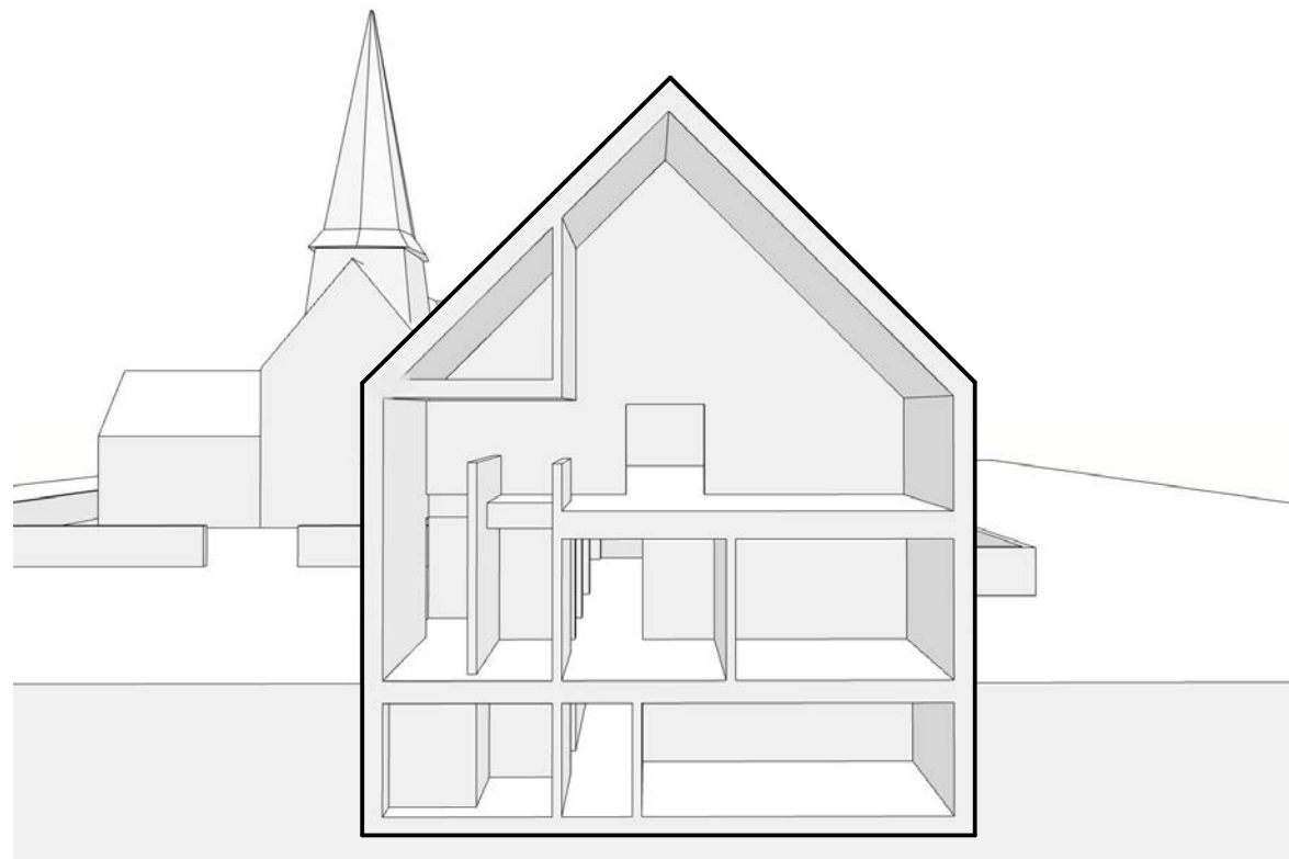
SCHNITT FOYER
